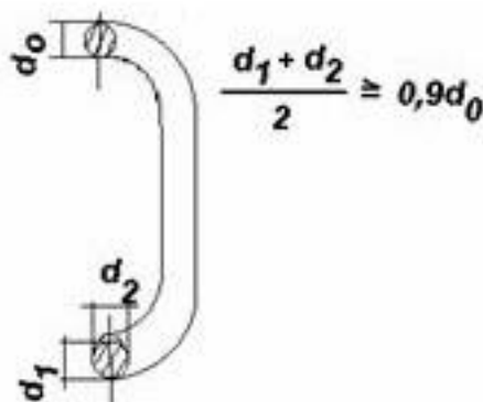
Рис. 2. Уменьшение диаметра сечения звена цепи:
