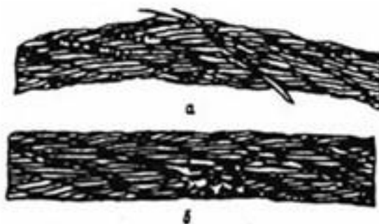
Рис. 3. Обрывы проволок в зоне уравнивающего блока:
