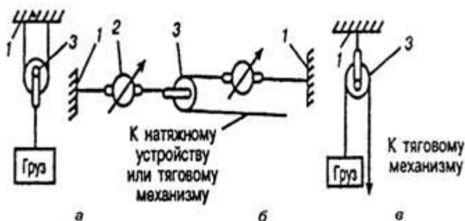
Рисунок 4.3. Схема испытания однорольных блоков:
