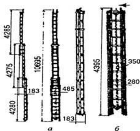
Рисунок 5.1. Условное изображение приставной раздвижной лестницы Л-3К:
