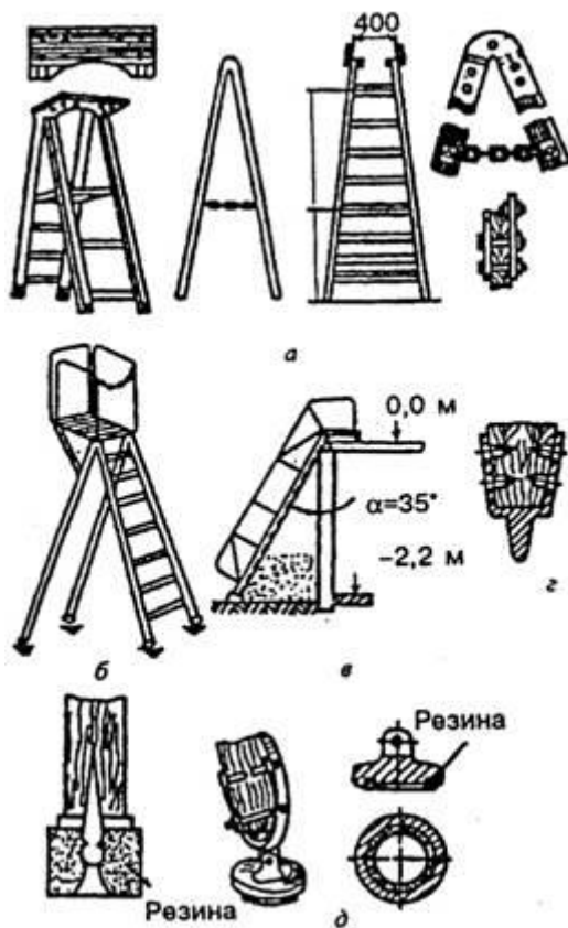
Рисунок 5.3. Стремянки а - деревянные; б - металлическая; в - трап для спуска в котлован;
