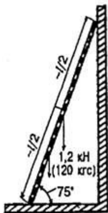
Рисунок 5.5. Схема испытания приставной лестницы.
