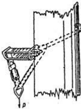
Рисунок 6.1. Схема испытания монтерских когтей: (Р - испытательная нагрузка)
