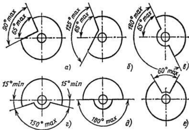
Рисунок 3.1. Расположение и наибольшие допустимые углы раскрытия защитных кожухов:
