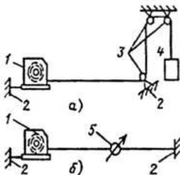
Рисунок 4.1. Схема испытания лебедок:
