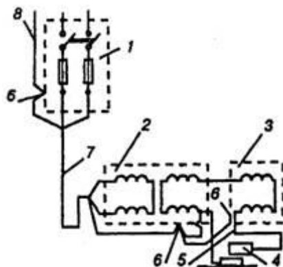
Рисунок 7.1. Схема подключения сварочного трансформатора:
