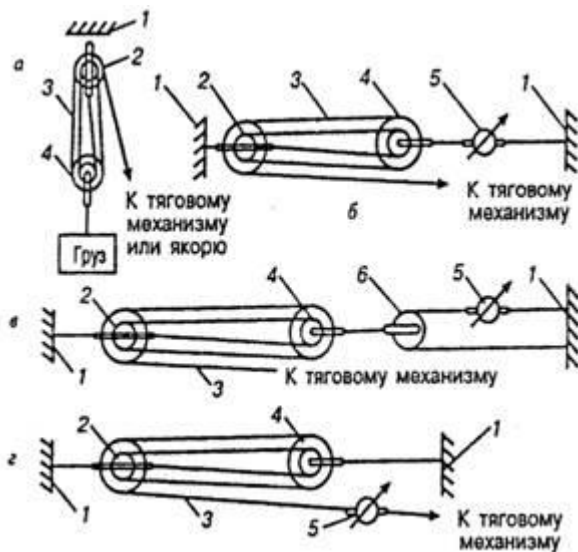
Рисунок 4.4. Схема испытания многорольных блоков и полиспастов:
