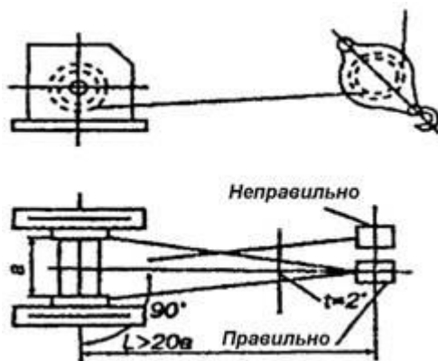
Рисунок 4.2. Намотка каната на барабан.
